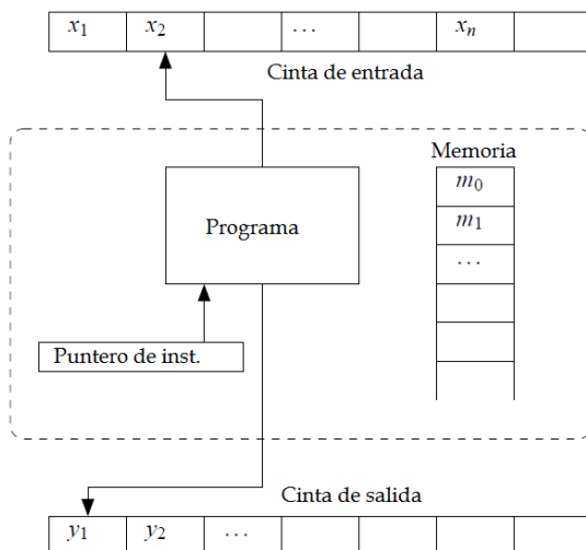
Figura 2.1: Máquina de acceso aleatorio (RAM).
